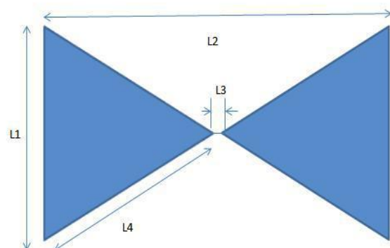
Fig 1:A simple Bow-Tie antenna
